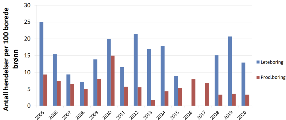
Figur 5-13 Brønnkontrollhendelser per 100 brønner, lete- og produksjonsboring, 2005-2020
