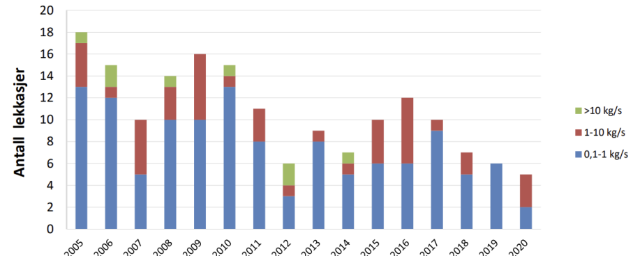
Figur 5-5 Antall lekkasjer, alle innretninger, norsk sokkel
